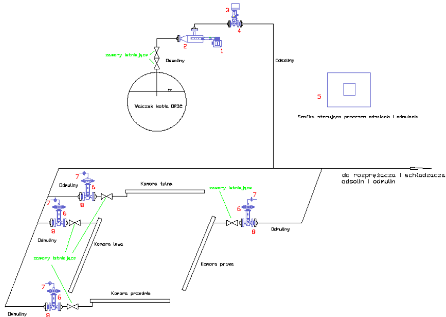
Rys. 14 Zakres modernizacji i automatyzacji systemu odsalania i odmulania na kotle wodnorurkowym
