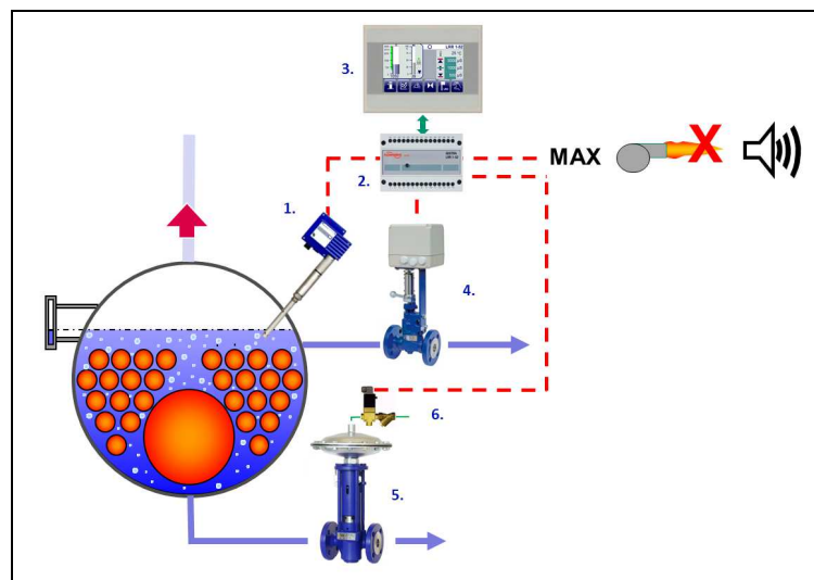
Rys 9. Elementy systemu automatycznego odsalania i odmulania kotła parowego
