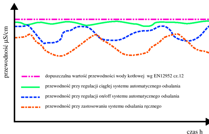
Rys 10. Zbliżenie przewodności wody kotłowej do wartości granicznej powoduje ograniczenie strumienia odsolin
