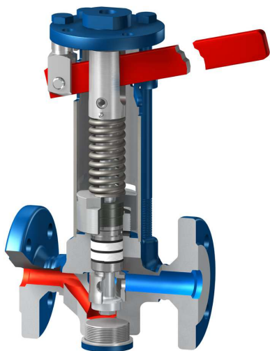
Rys 11. Zawór odmulający szybkozamykający PA/MPA 46/47 dla kotłów parowych
