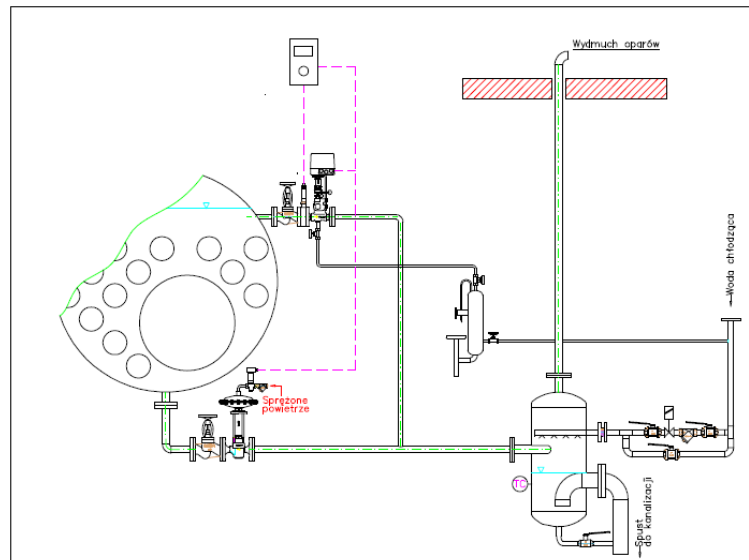
Rys. 16 Zakres modernizacji i automatyzacji systemu odsalania i odmulania na kotle płomienicowo-płomieniówkowym
