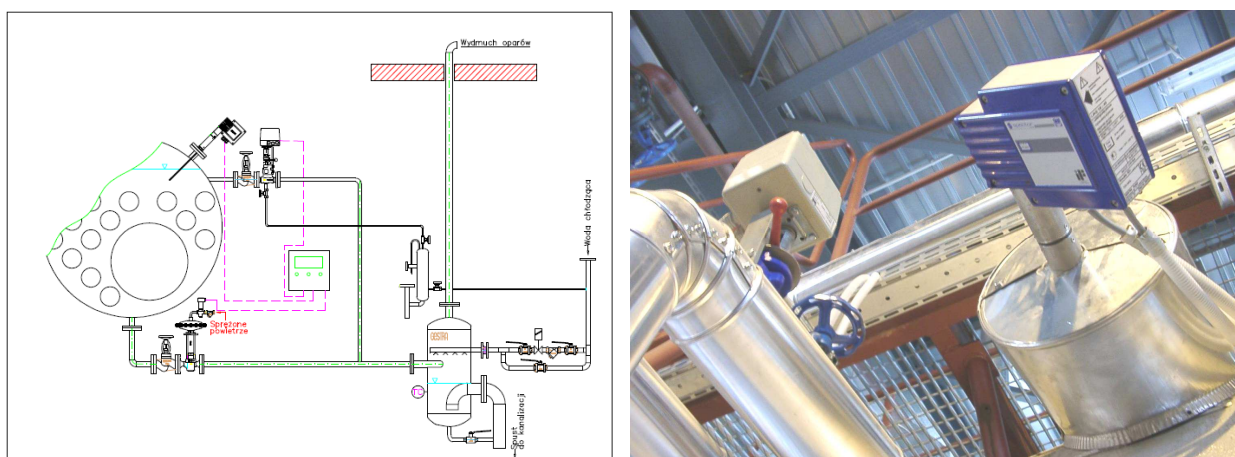
Rys. 13 Zalecany sposób instalacji elektrody z końcówką pomiarową wewnątrz walczaka kotła (kotły nowe <60bar)
