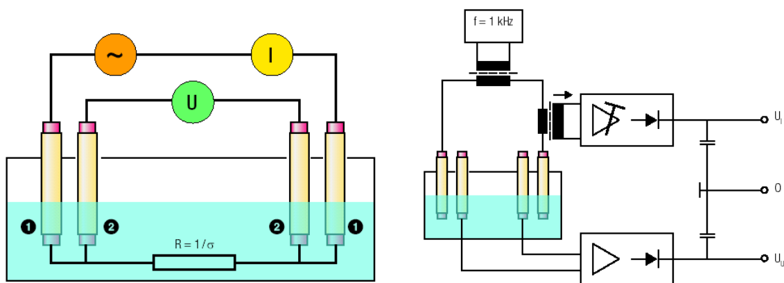
Rys 6. Zasada działania systemu czteroelektrodowego pomiaru przewodności wody
