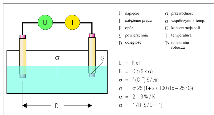
Rys. 2 Zasada pomiaru przewodności cieczy
