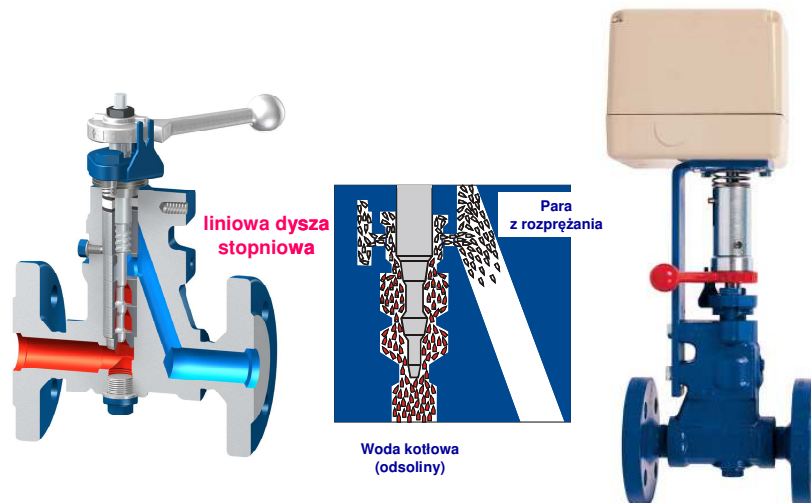
Rys 8. Zawór odsalający dla kotłów parowych z liniową dyszą stopniową typ BA/BAE 46/47
